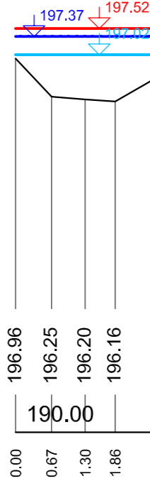
P 5 - 0.08000 km
