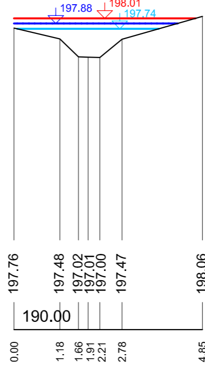
P 12 - 0.23100 km
