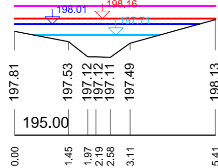
P 13 - 0.24000 km
