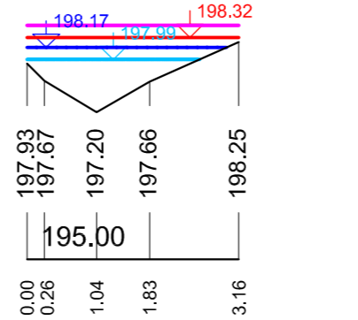
P 15 - 0.26600 km
