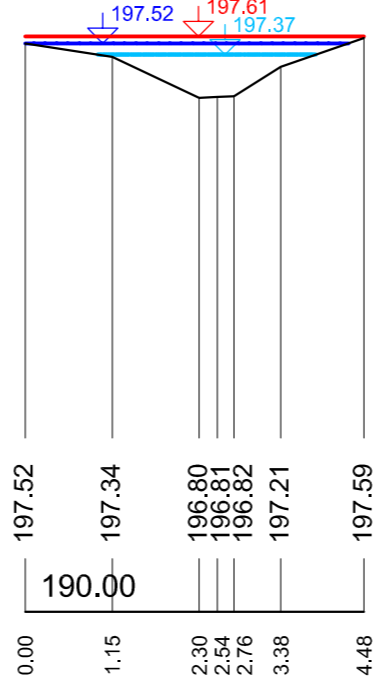
P 14 - 0.25200 km
