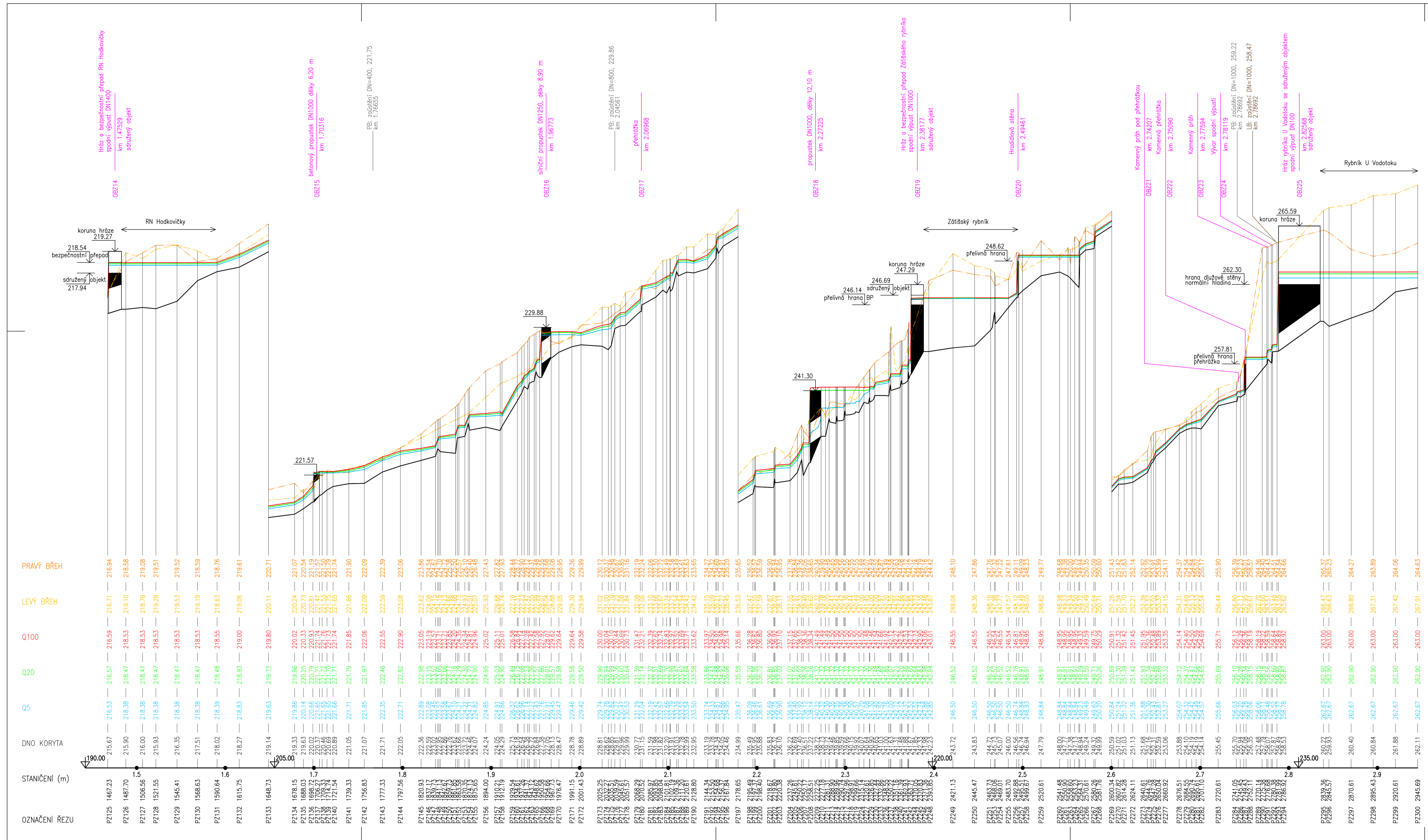
Podélný profil ZÁTIŠSKÝ POTOK: km 1.480 – 2.950 Měřítko 1 : 2000 / 100
