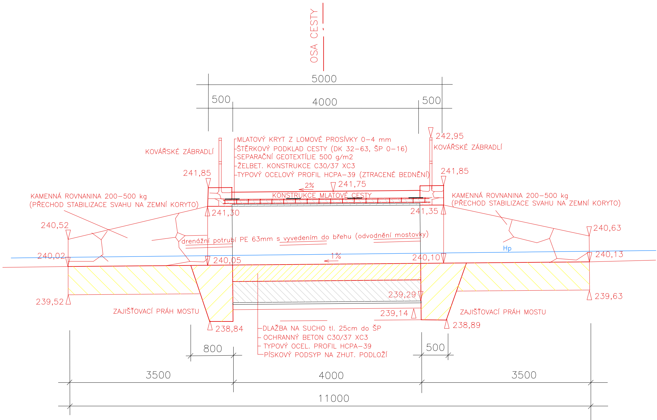
D.2.11 PODÉLNÝ PROFIL MOSTKEM v měř. 1 : 50
